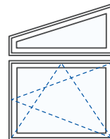
INNADSLÅENDE VINDU MED FAST OVERFELT MED SKRÅKARM** Maksmål: 1.500 (b) 2.700 (h)
